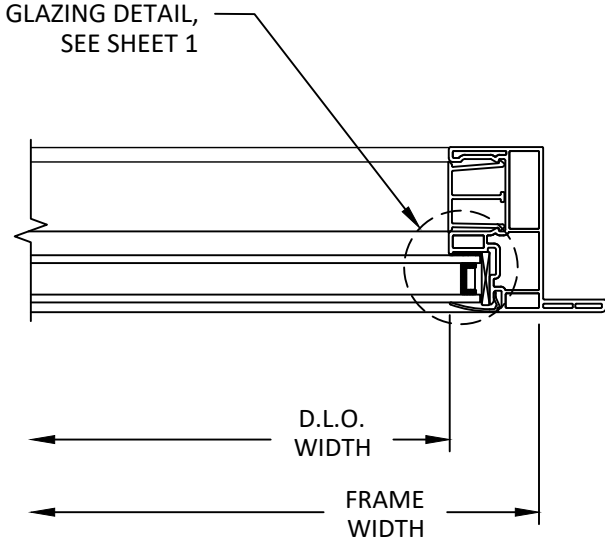
B 5 HORIZONTAL SECTION V152 JAMB
