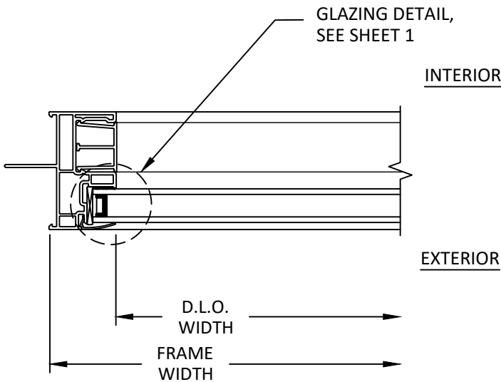
C 5 HORIZONTAL SECTION V100 JAMB
