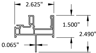
2 V100 FRAME HEAD/SILL/JAMB
