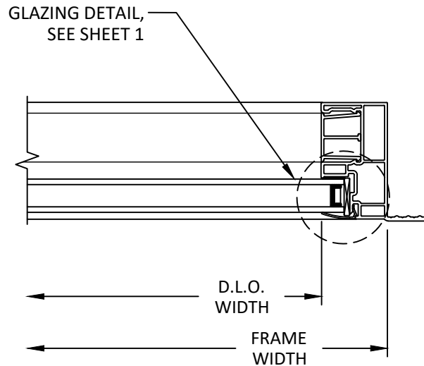
D 5 HORIZONTAL SECTION V101 JAMB
