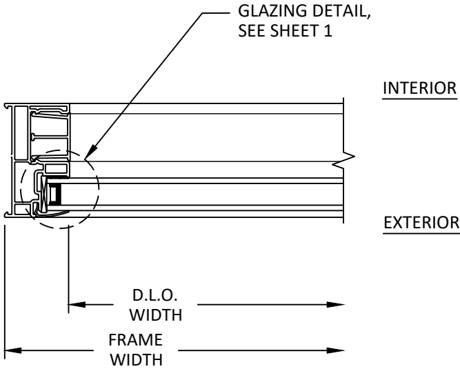
A 5 HORIZONTAL SECTION V142 JAMB
